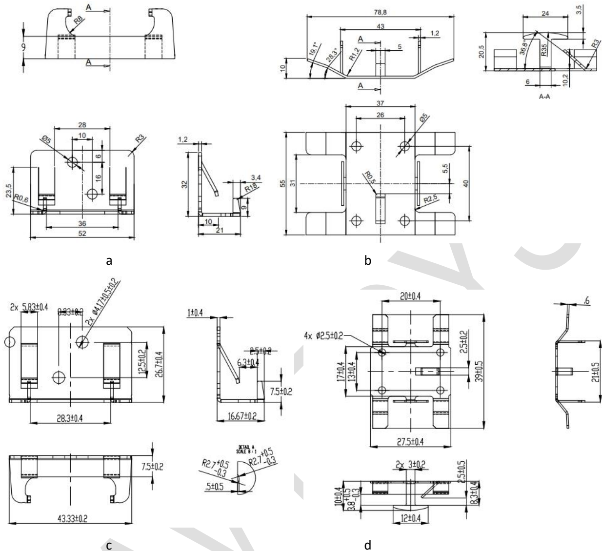
4 pav. – tvirtinimo elementai apdailinėms plytelėms (kabliukai): pirmo tipo kabliukai – a (viengubi) ir b (dvigubi); antro tipo kabliukai – c (viengubi) ir d (dvigubi)
